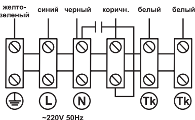
Схема подключения №4
