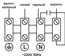
Схема подключения №3
