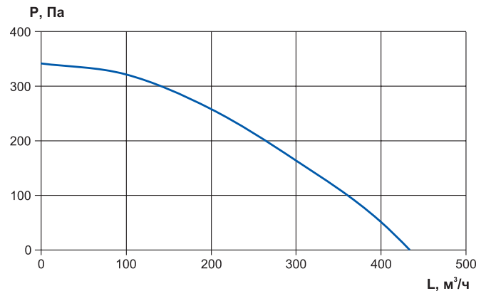
CV-SH-200-AC
