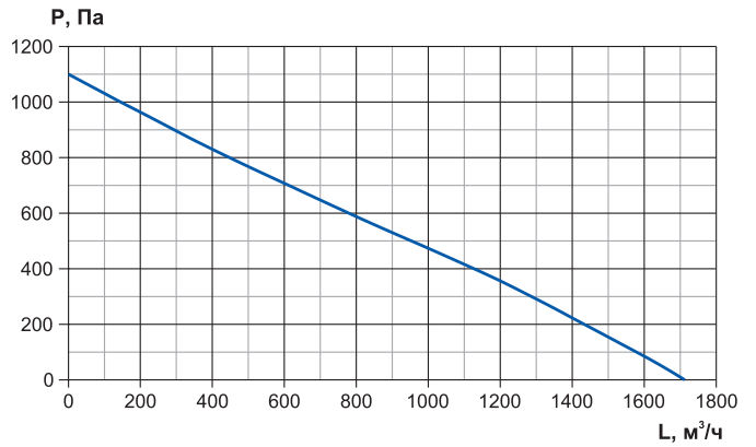
RWN-RP-2000-EC-Vertical-Aqua
