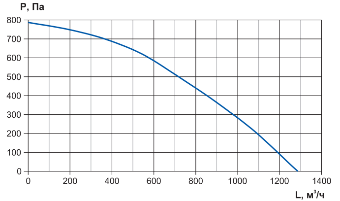
RWN-RP-1600-EC-Vertical-Aqua
