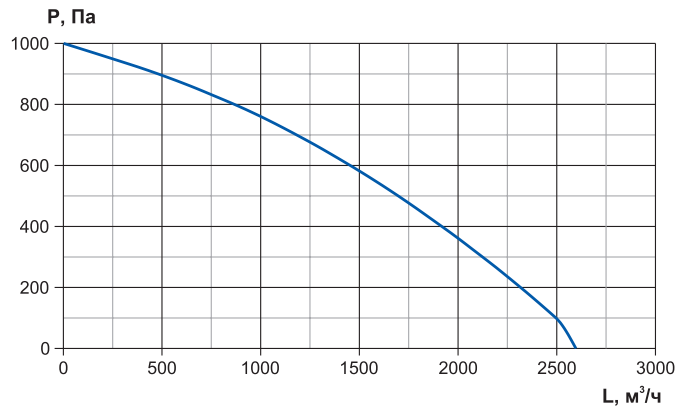
RWN-RP-2500-EC-Vertical-Aqua
