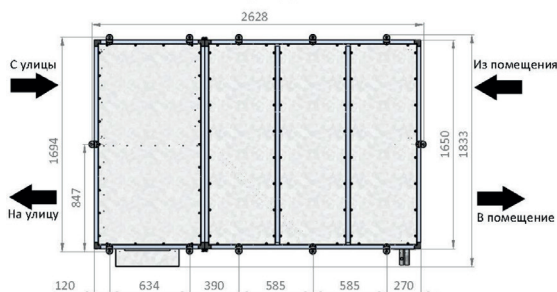
Вид сверху
