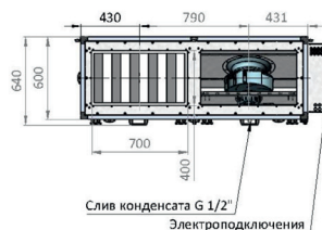
Вид слева
