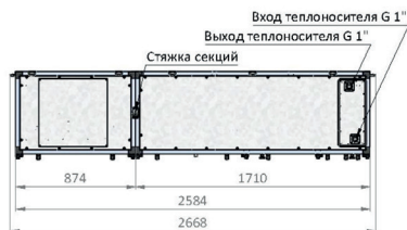
Вид спереди
