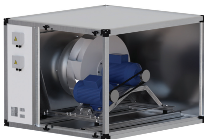
Вентилятор с резервным двигателем
